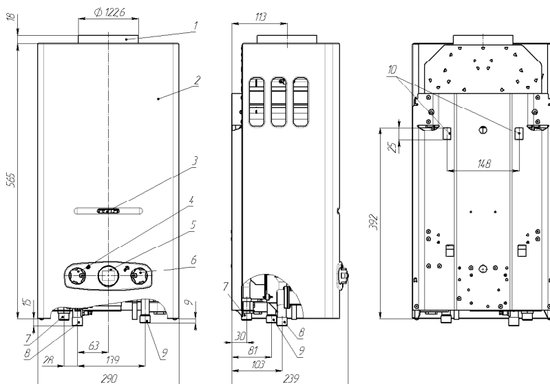
а) МАКТЕРМ Стандарт 10, МАКТЕРМ Стандарт 11
