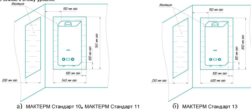
Рисунок 2. Пример установки аппаратов на труднোগреемых стенах
