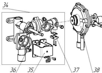
Рисунок 9. Узел водогазовый
