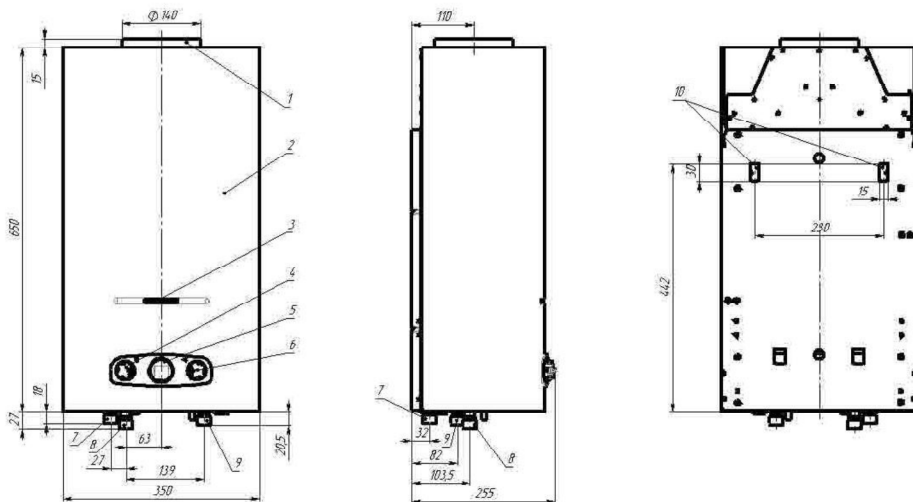
б) МАКТЕРМ Стандарт 13
