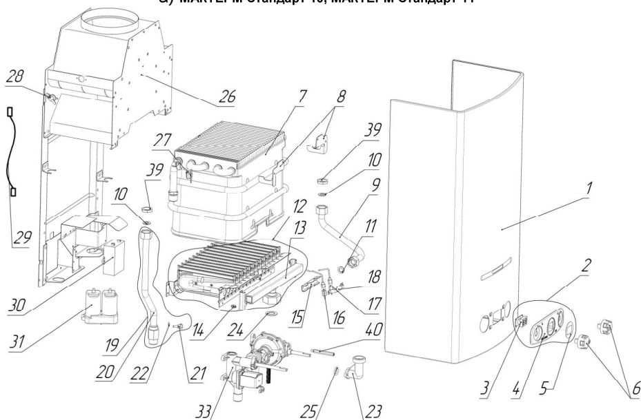
б) МАКТЕРМ Стандарт 13
